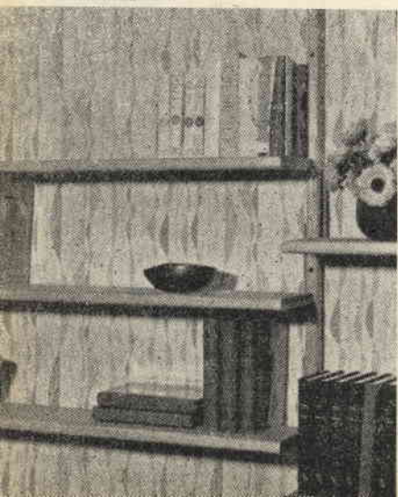
◀ Fig. 37 - Montanti e ripiani in quercia lucidata. Fissaggio dei montanti alla parete a mezzo 3 viti. Larghezza frontale ripiani mm. 800, profondità mm. 160. Altezza montanti mm. 1000; distanza fra i ripiani regolabile con salti di 50 millimetri.
