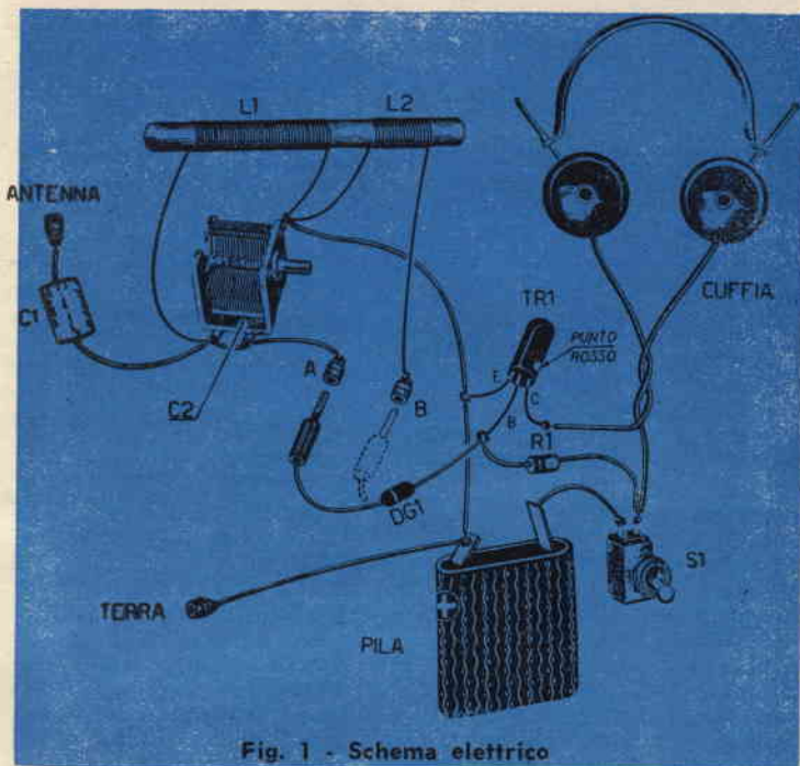
Fig. 1 - Schema elettrico
