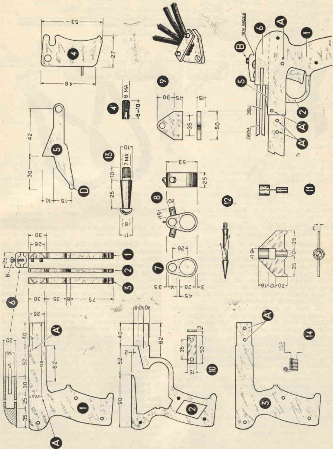
Fig. 1 - Dimensionamento particolari.
