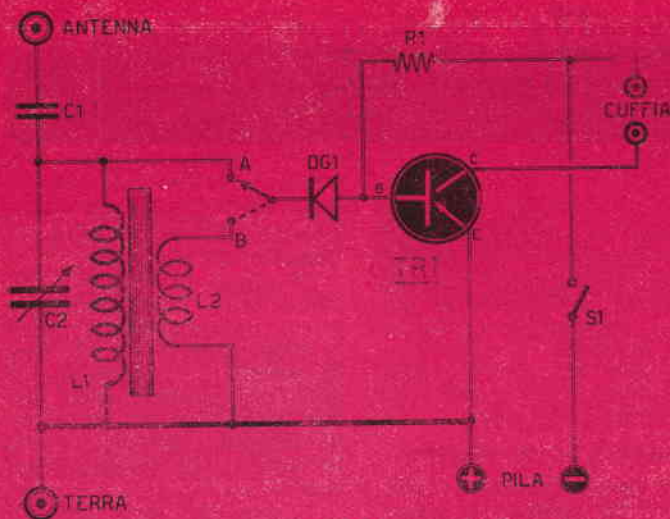
Fig. 2 - Schema pratico.
