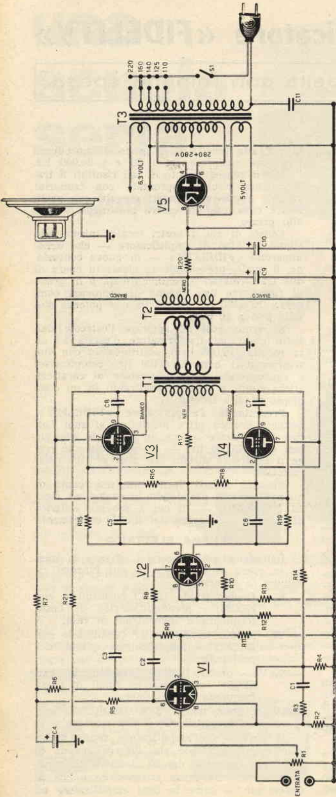
Fig. 1 - SCHEMA ELETRICO
