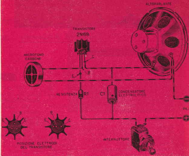
Fig. 3 - Schema pratico
